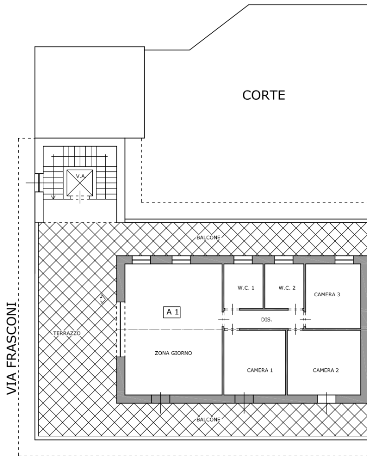
VIA CUSTODI PIANO SOTTOTETTO tipo 1
