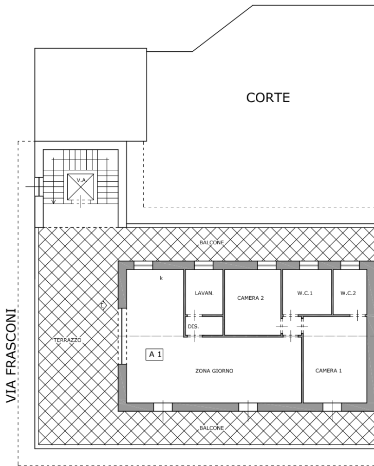
VIA CUSTODI PIANO SOTTOTETTO tipo 5
