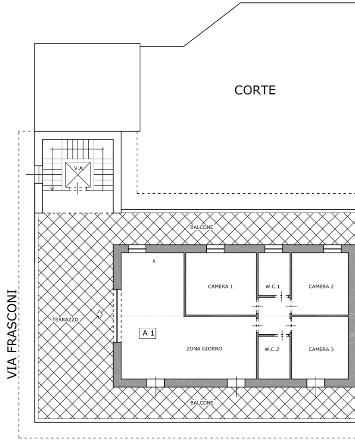
VIA CUSTODI PIANO SOTTOTETTO tipo 10
